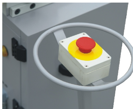
Giętarka - urządzenie elektryczne do wyginania łuków, kątów w rurach i szynach
